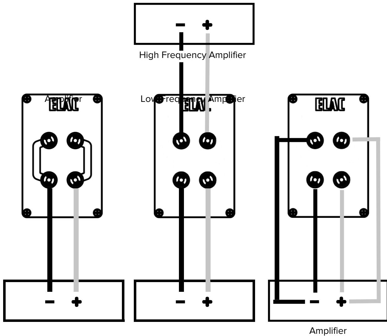
Fig. 1—Single Wiring
