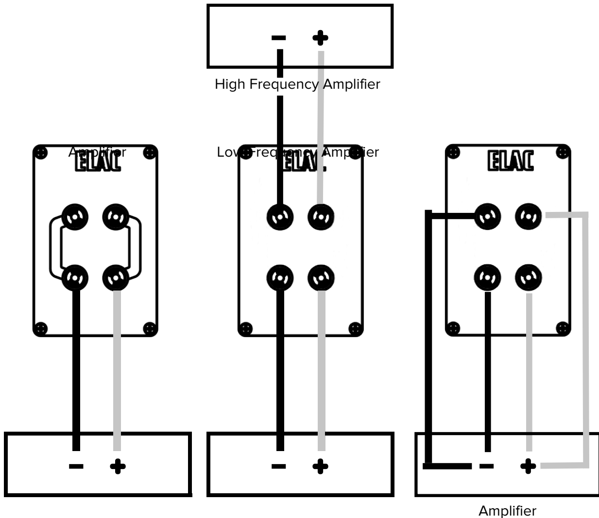
Fig. 1—Single Wiring
