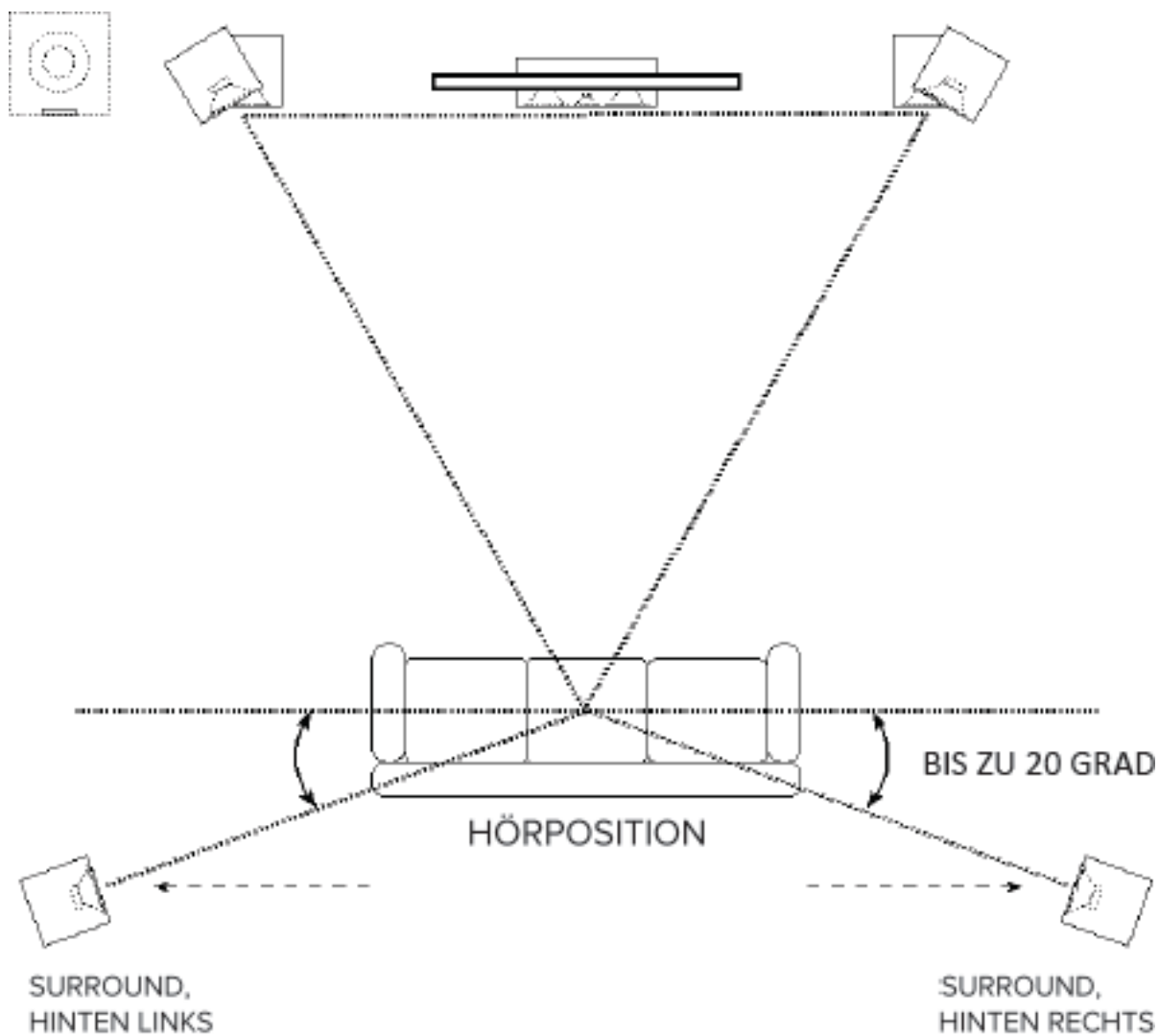
5.1 KANAL-SURROUND-KONFIGURATION
